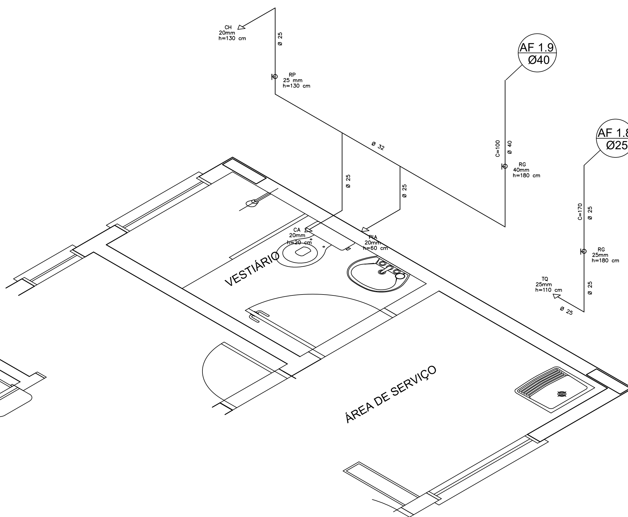
5 ÁREA DE SERVIÇO E VESTIÁRIO - ESQUEMA ISOMÉTRICO ESCALA 1/25
