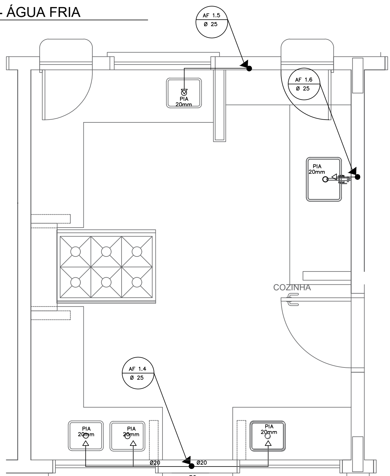
2 COZINHA - PLANTA BAIXA ESCALA 1/25
