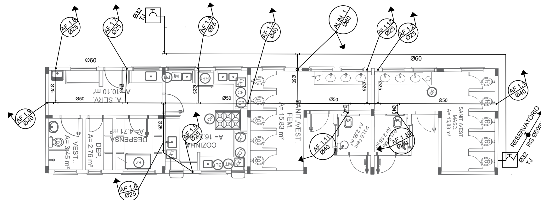
1 PLANTA BAIXA - ÁGUA FRIA ESCALA - 1:100
