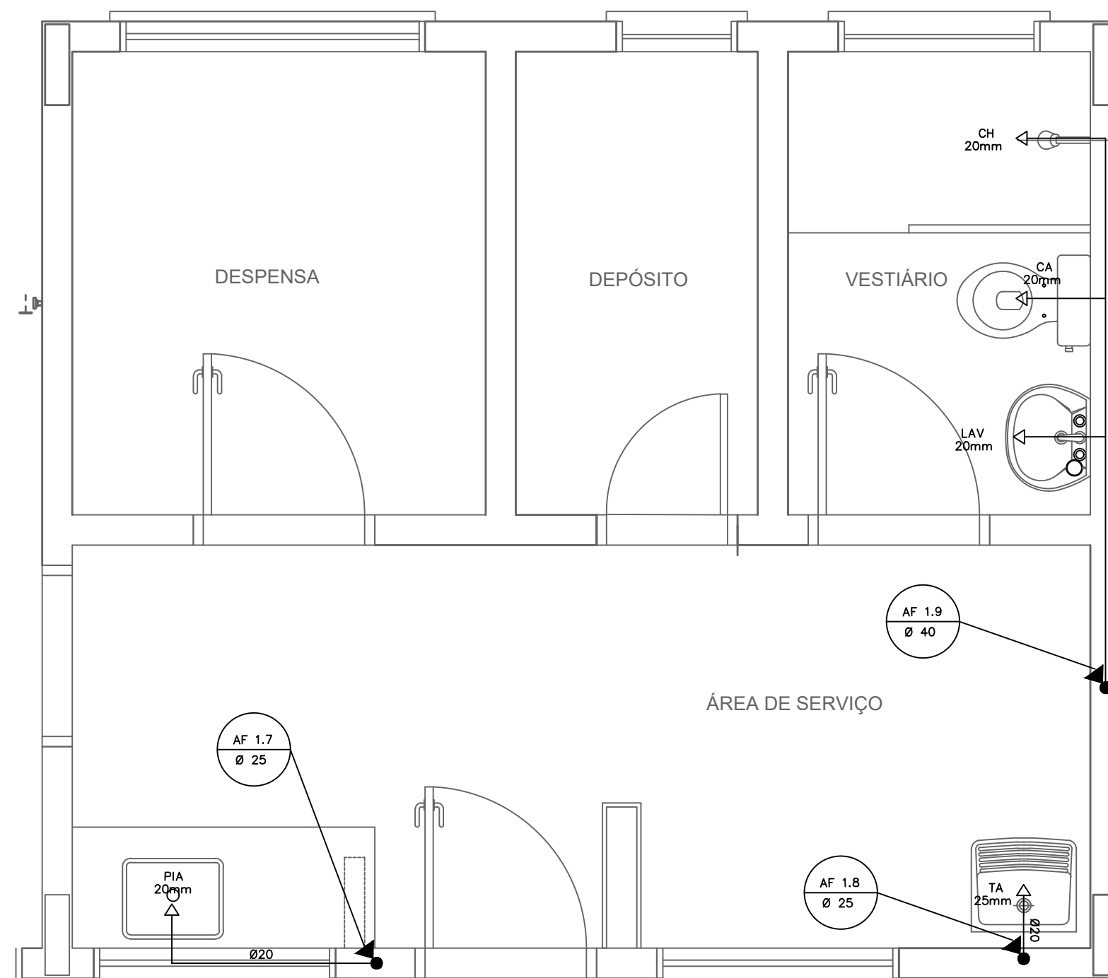
4 ÁREA DE SERVIÇO E VESTIÁRIO - PLANTA BAIXA ESCALA 1/25
