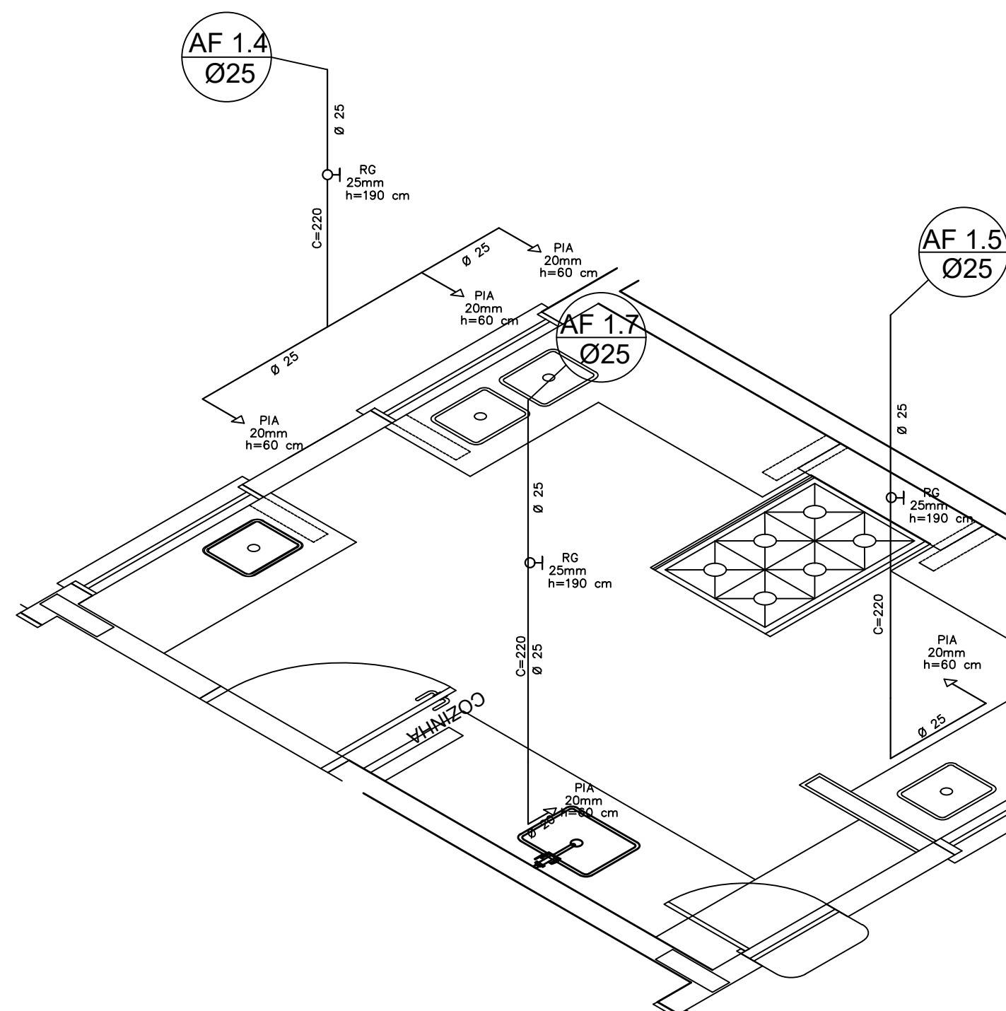
3 COZINHA - ESQUEMA ISOMÉTRICO ESCALA 1/25
